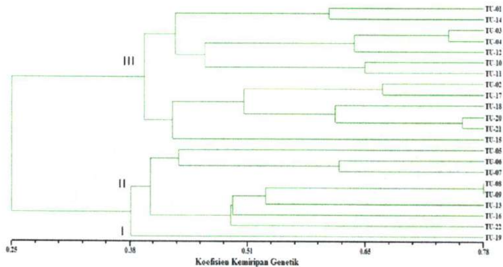
Gambar 3. Hasil analisis kluster 22 aksesori padi lokal Toraja Utara berdasarkan 26 marka SSR menggunakan program NTSYS pc 2.1
